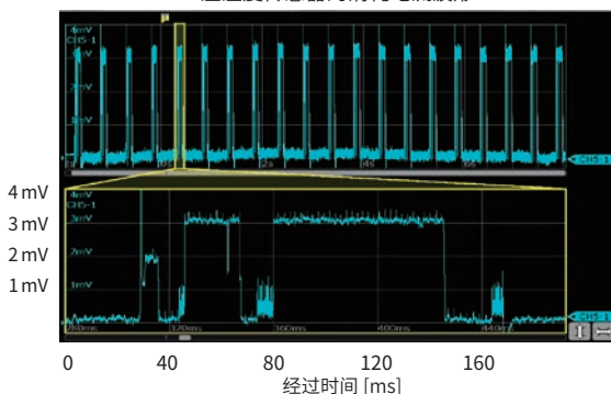
用CT6711 (10V/A 量程) 测量时
