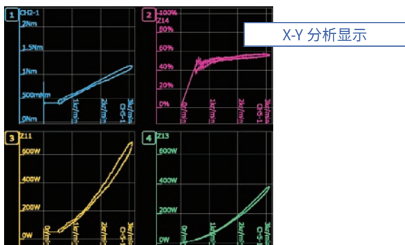
支持 4 画面的 X-Y 显示
