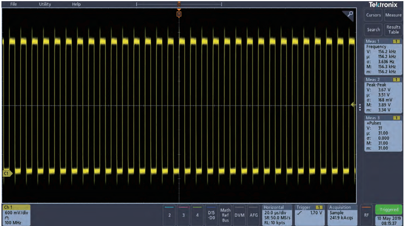
自动测量频率、峰峰值和正脉冲数，并显示统计数据。
