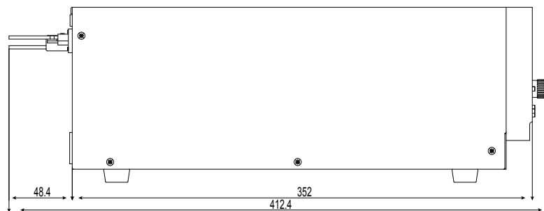
侧视图
