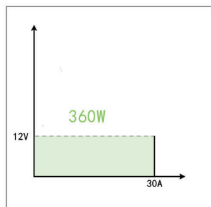
传统矩形输出模式，固定量程12V30A
