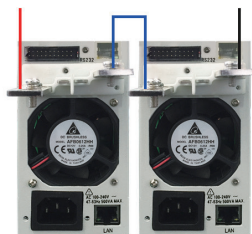
两台串联工作
