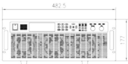
正视图
