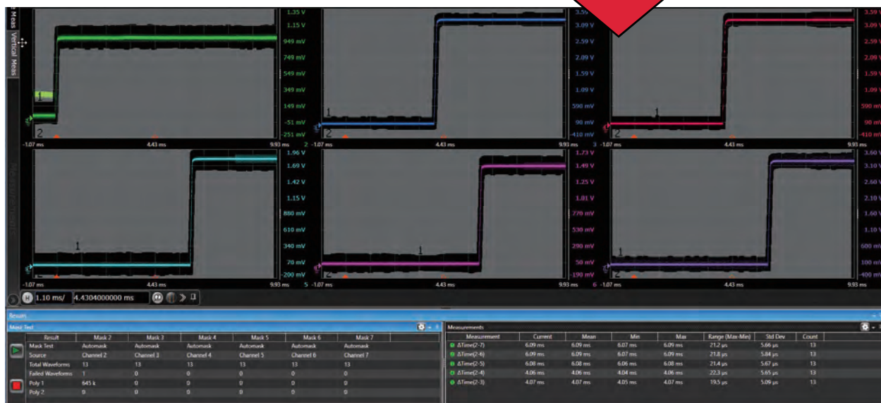
通过将不同通道波形放置于不同网格并进行独立的模板测试，您可以在成千上万个启动周期中对这六个电源轨进行连续测试。
